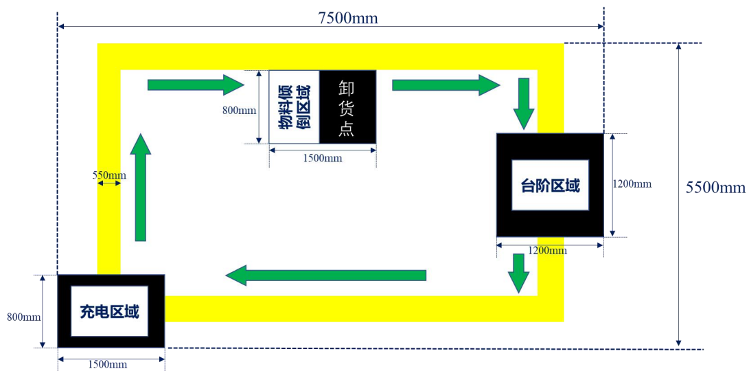
图 1-区域（省）选拔赛场场地平面参考图
